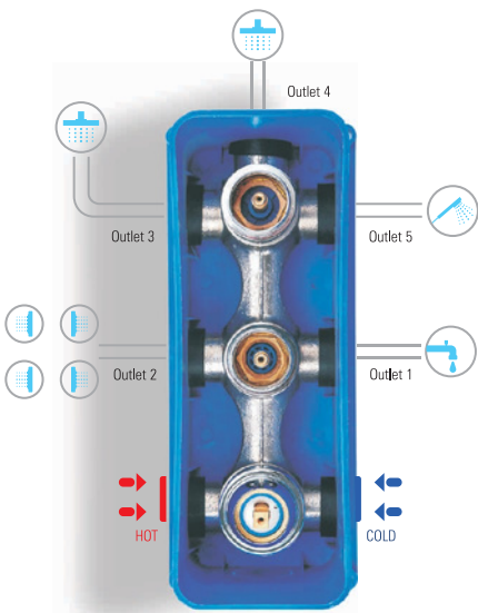
DCB 4025 MRP ₹ 17350/- (Chrome)
